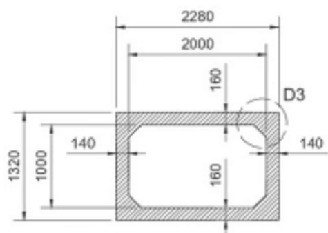
SECCIÓN ALCANTARILLA ENCOFRADO
