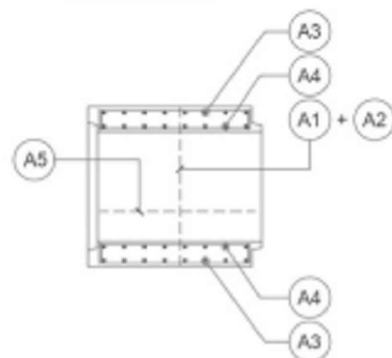
PLANTA ALCANTARILLA ARMADURA
