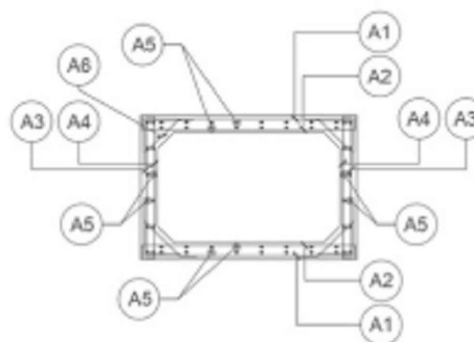
SECCIÓN ALCANTARILLA ARMADURA
