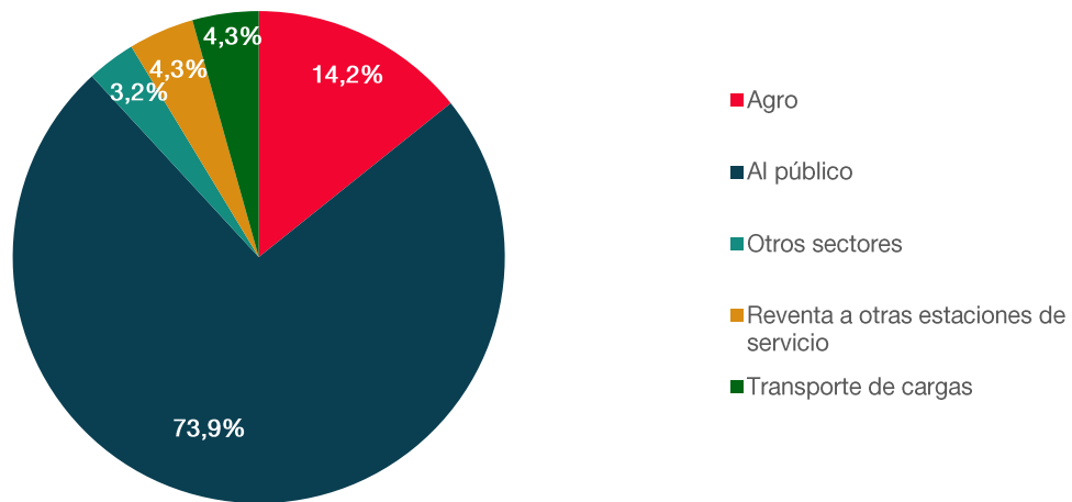
Gráfico N° 6: Porcentaje de metros cúbicos de gasoil grado 3 comercializados según canal de comercialización. Municipio de Crespo. Acumulado a diciembre 2024.
