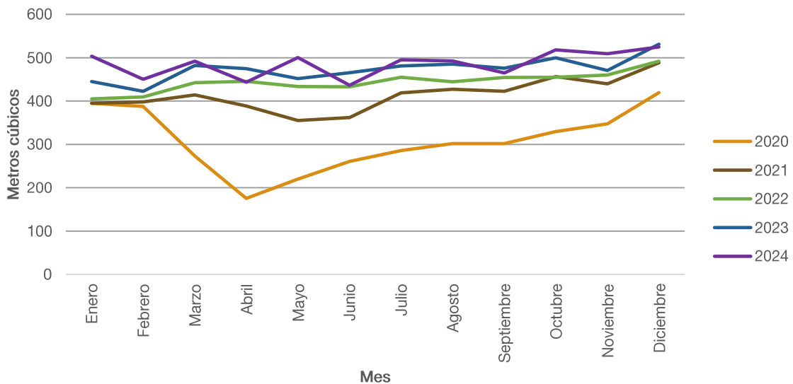
Gráfico N° 7: Metros cúbicos de nafta súper (entre 93 y 95 ron) comercializados por mes. Municipio de Crespo. Años 2020-2024
