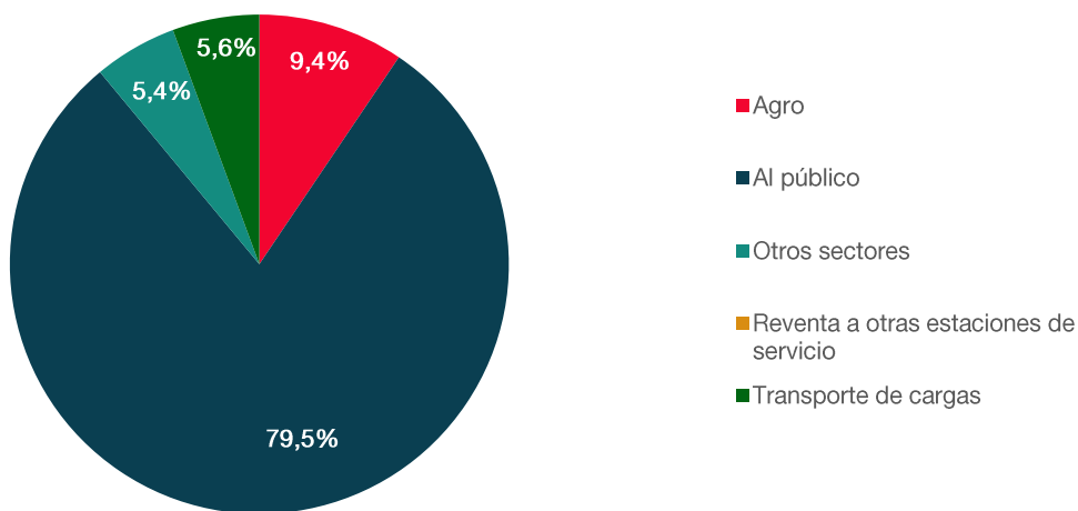
Gráfico N° 5: Porcentaje de metros cúbicos de gasoil grado 3 comercializados según canal de comercialización. Municipio de Crespo. Diciembre 2024.
