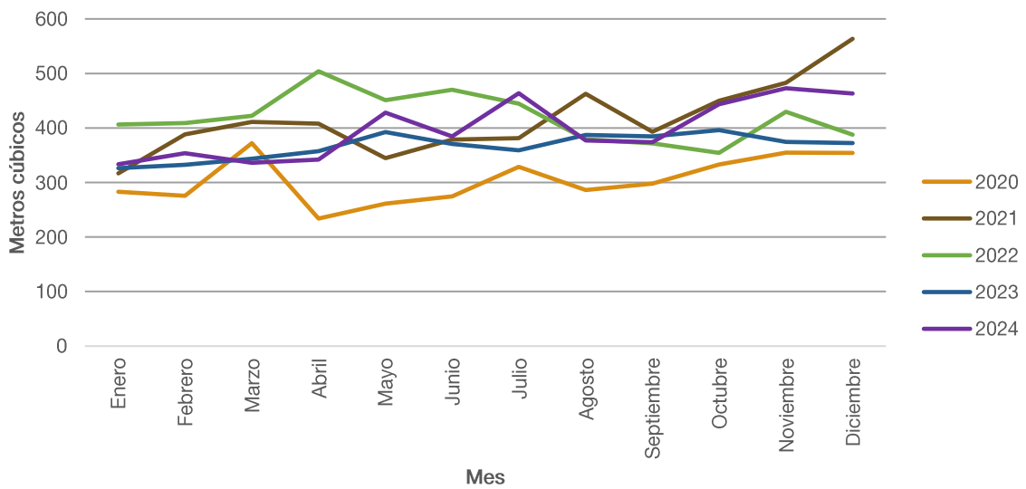
Gráfico N° 4: Metros cúbicos de gasoil grado 3 comercializados por mes. Municipio de Crespo. Años 2020-2024
