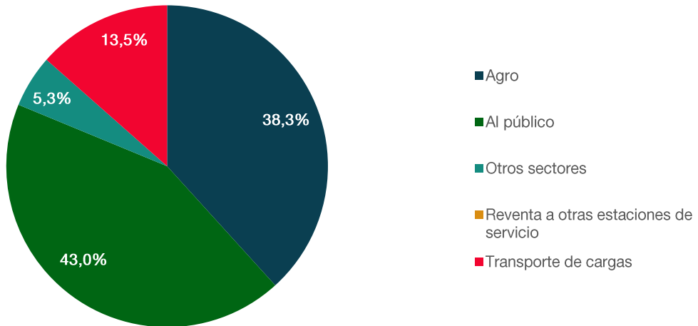
Gráfico N° 2: Porcentaje de metros cúbicos de gasoil grado 2 comercializados según canal de comercialización. Municipio de Crespo. Diciembre 2024.
