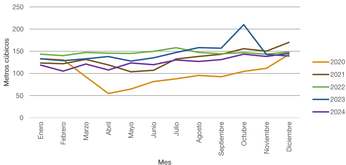
Gráfico N° 8: Metros cúbicos de nafta premium (más de 95 ron) comercializados por mes. Municipio de Crespo. Años 2020-2024
