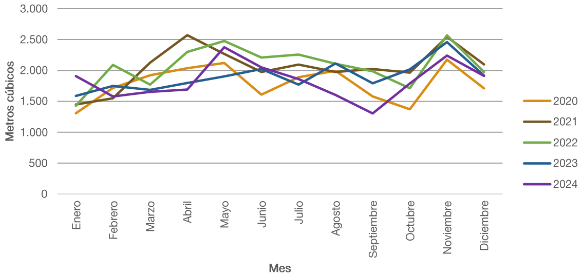
Gráfico N° 1: Metros cúbicos de gasoil grado 2 comercializados por mes. Municipio de Crespo. Años 2020-2024
