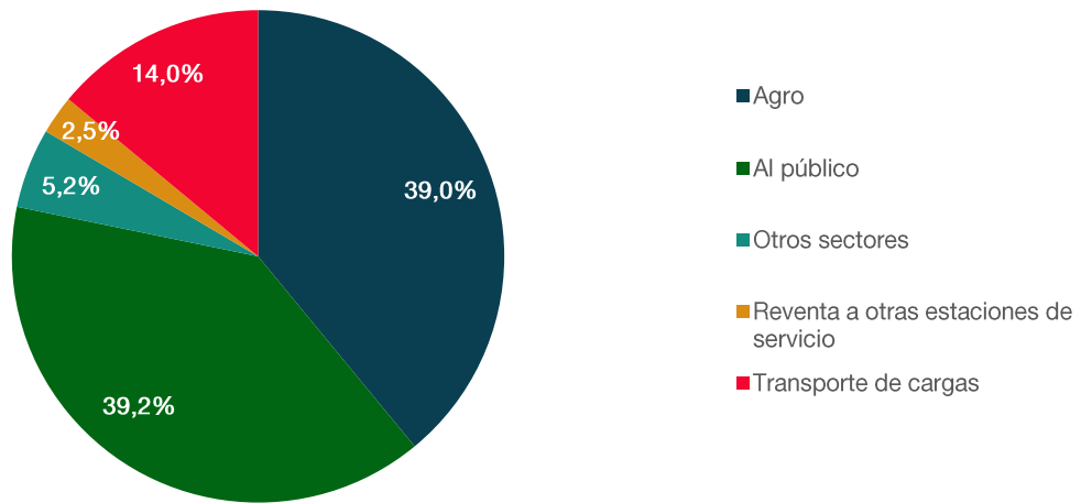
Gráfico N° 3: Porcentaje de metros cúbicos de gasoil grado 2 comercializados según canal de comercialización. Municipio de Crespo. Acumulado a diciembre de 2024.
