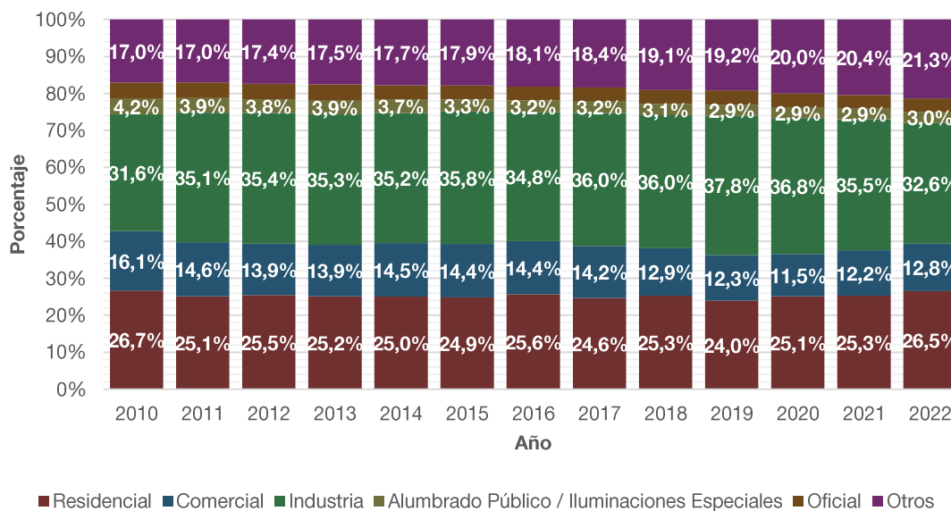
Gráfico N° 4.4.1.2.2: Participación porcentual de consumo de energía eléctrica según categoría de usuario. Municipio de Crespo. Años 2010-2022
